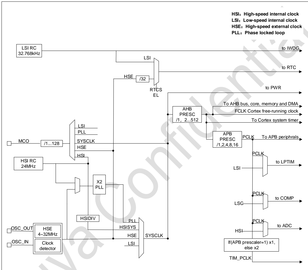
图 2-1 系统时钟结构图
