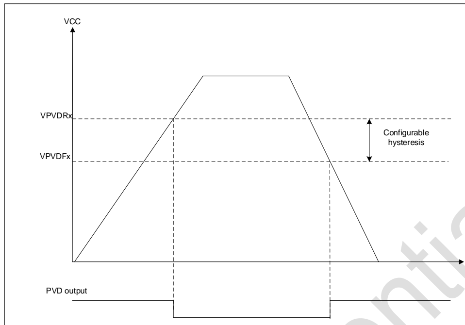
图 2-4 PVD 阈值
