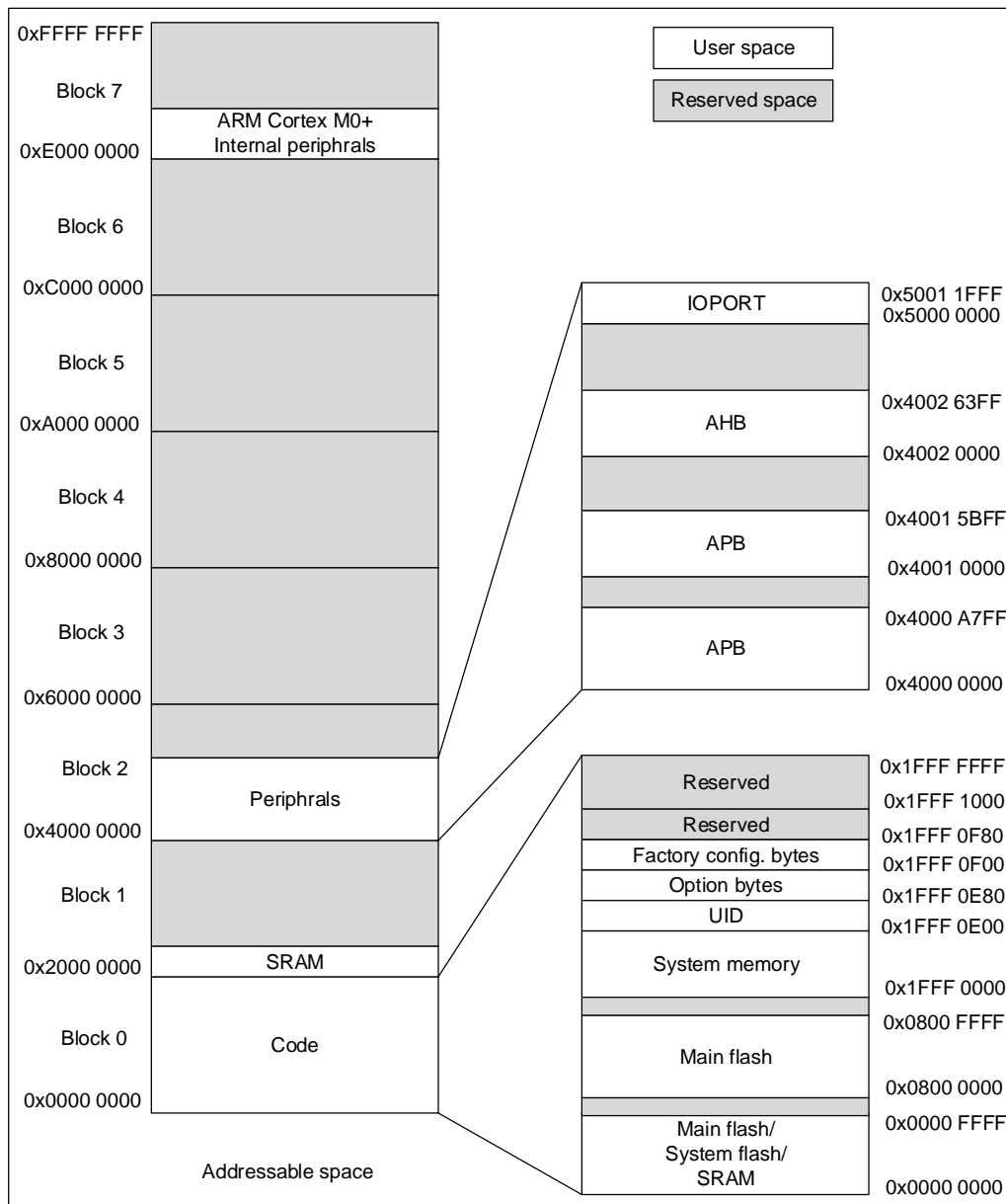
图 4-1 存储器映射
