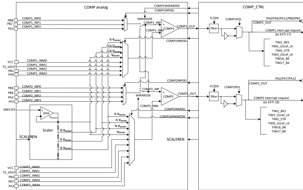
图 2-5 COMP 框图
