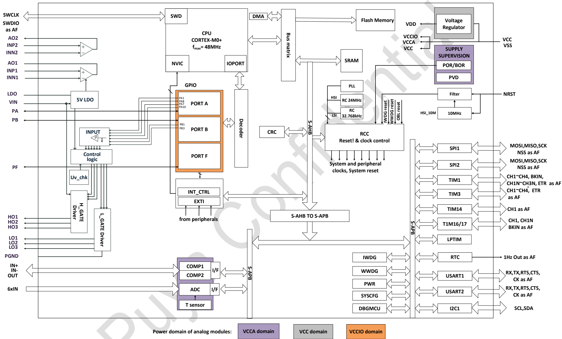
图 1-1 功能模块
